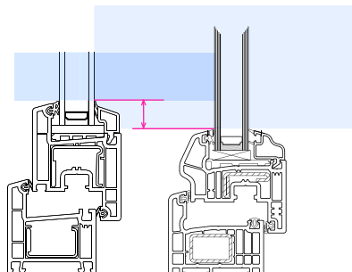
Обычное пластиковое окно
